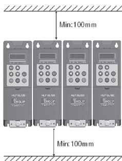
图2 并排安装
