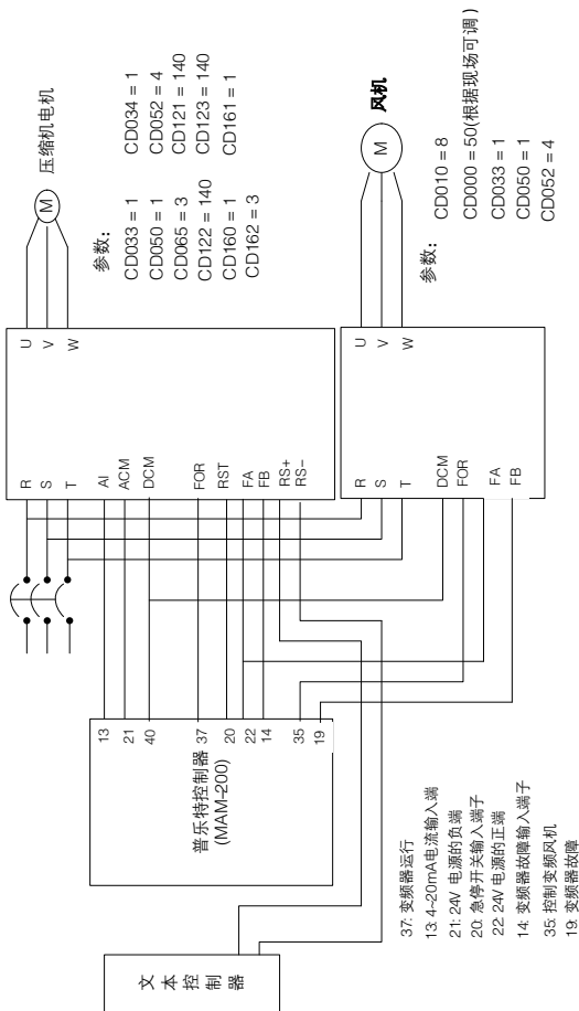
变频器与普乐特控制器(MAM200)的空压机应用案例
