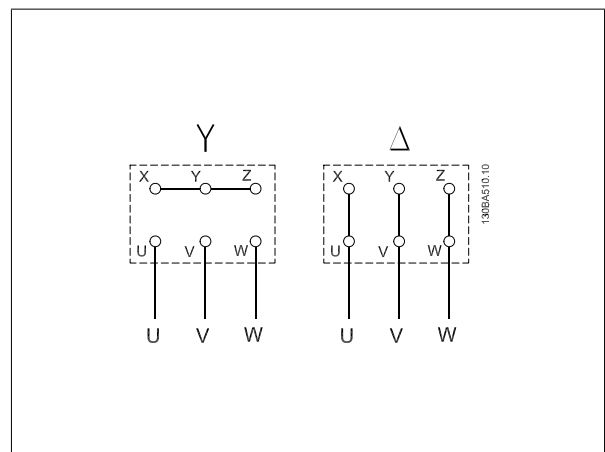
图 3.3: 星形和三角形连接。
