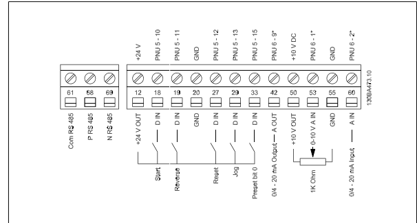
图 3.7: PNP 配置和出厂设置中的控制端子概述。
