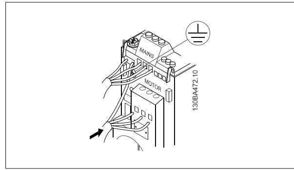
图 3.4: 安装接地电缆和电动机电线。
