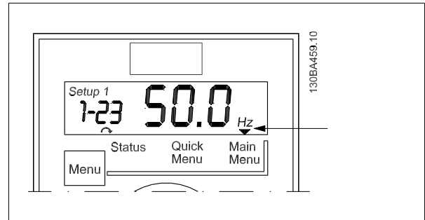
图 4.10: 指示主菜单模式
