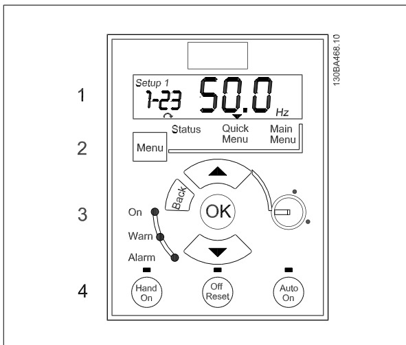
图 4.1: 带有电位计的 LCP 12
