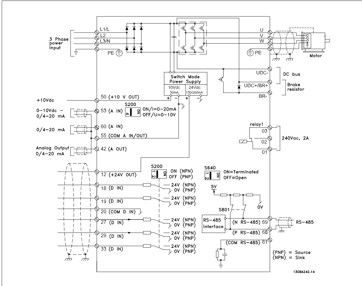
图 3.10: 图示显示了所有电气端子。
