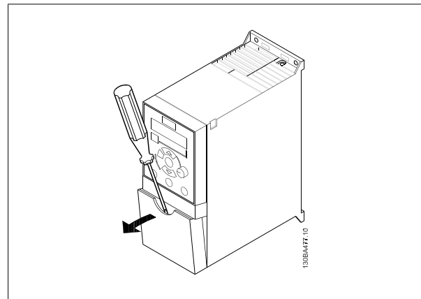
图 3.6: 取下端子盖。
