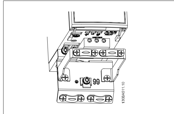
图 3.5: 带去耦板的 VLT Micro Drive
