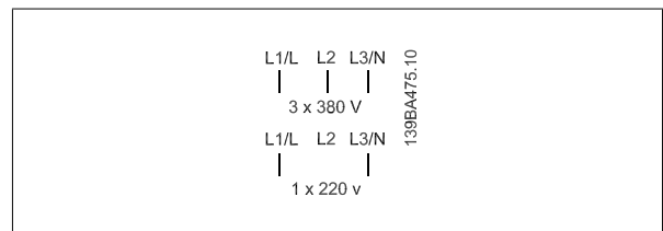
图 3.2: 三相和单相接线。
