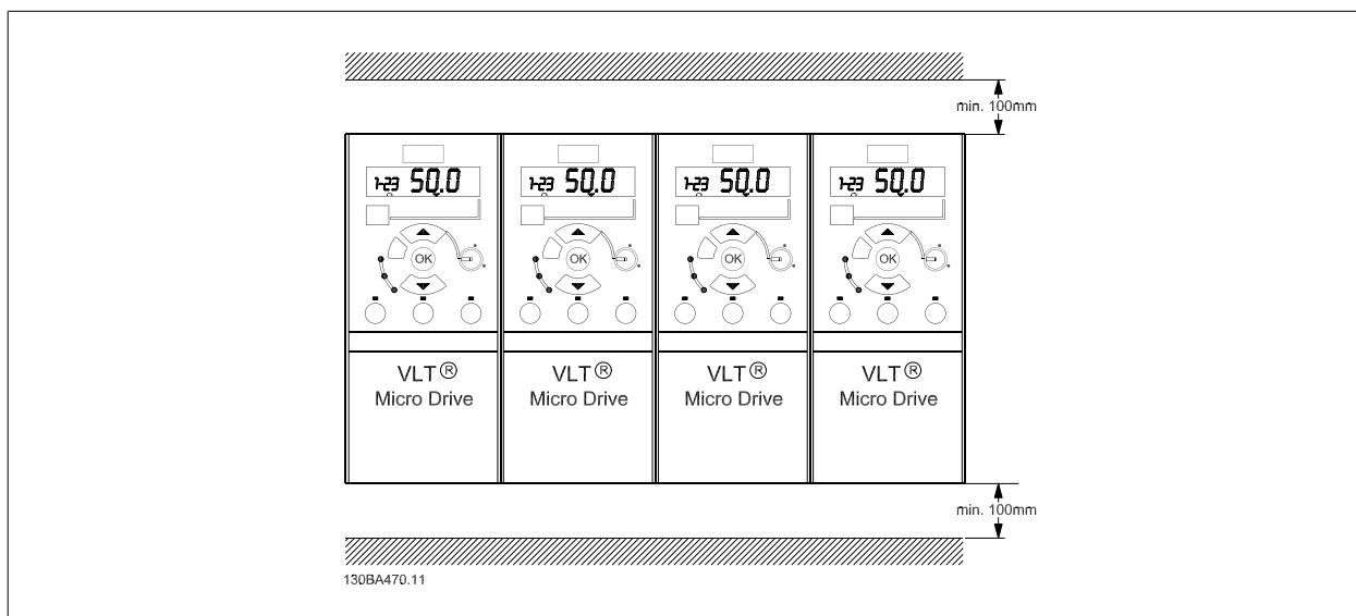
图 2.2: 并排安装。
