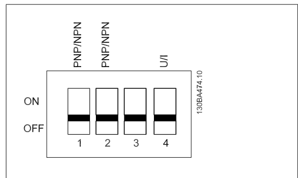
图 3.9: S200 开关 1-4
