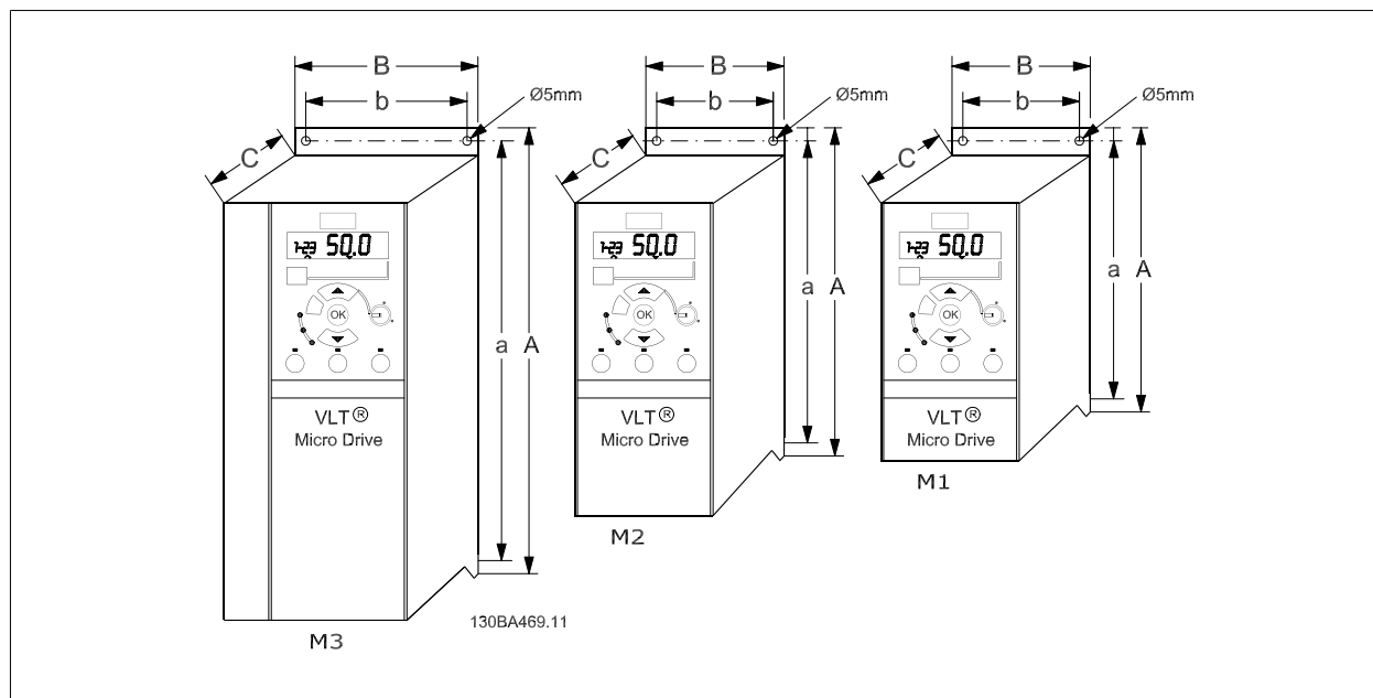
图 2.3: 机械尺寸。
