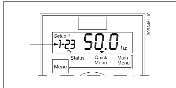
图 4.4: 指示选定的参数号
