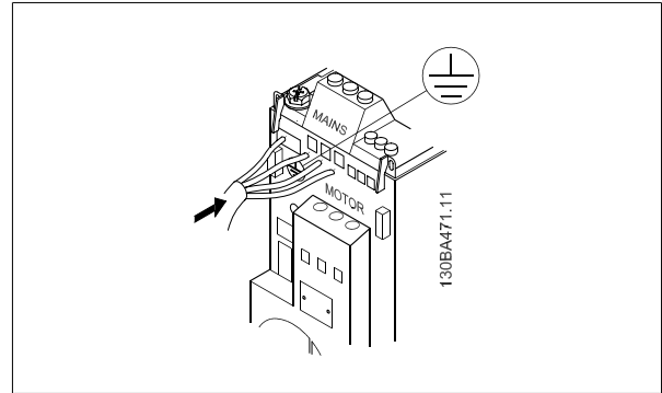
图 3.1: 安装接地电缆和主电源线。
