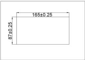
开孔尺寸
